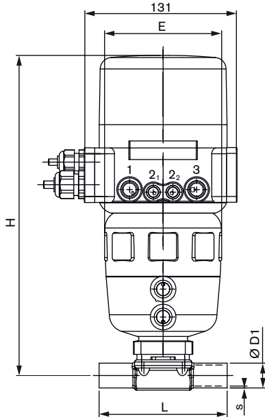
DN 15-50
